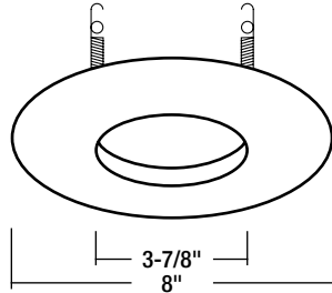
Trim OD: 8" Aperture: 3-7/8"
